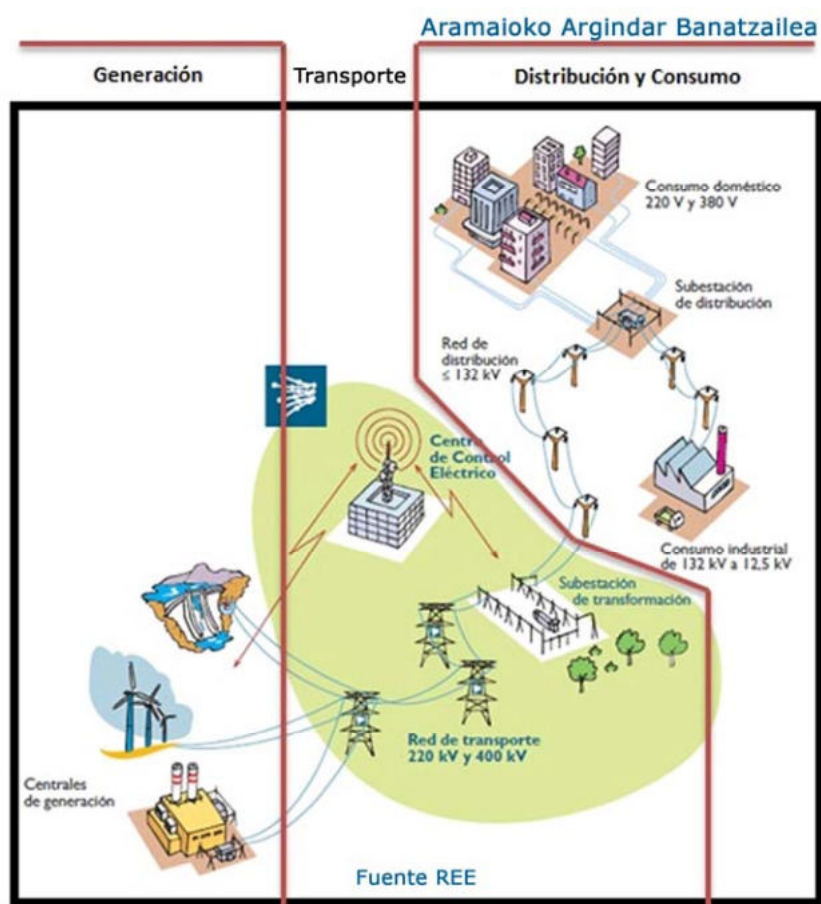
Elektrizitate banaketaren eskema
